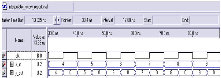
Fig. 10. Interpolator Output
